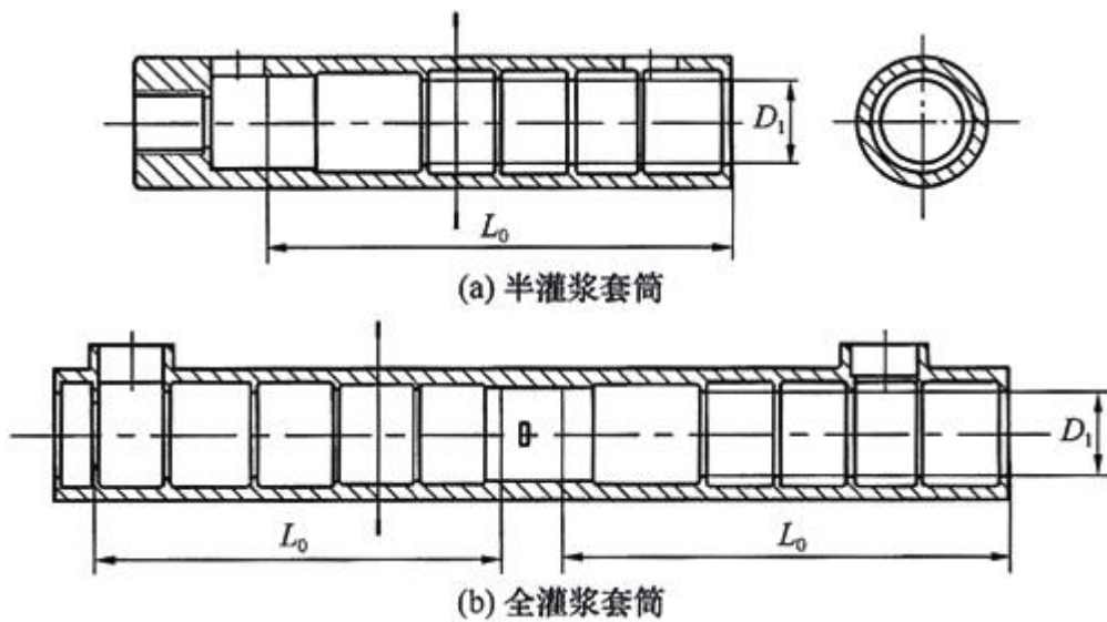
图 1 灌浆套筒示意
